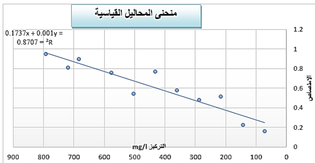
الشكل: (1) يوضح المنحنى القياسي لسلسلة المعايرة القياسية
